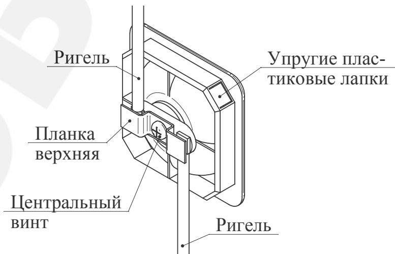
Рис. 8 Замок ригельный (Вид сзади)
