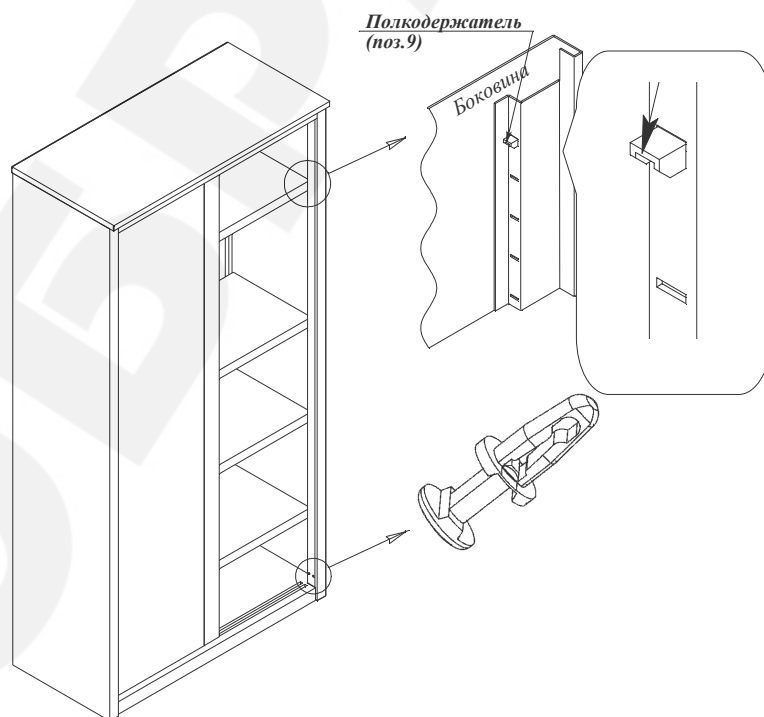
Рис.7а. Шкафы серии AL и ALS
