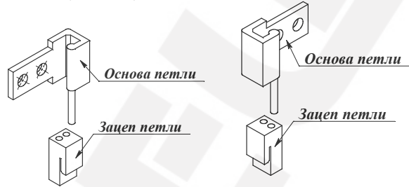
Петля правая (поз.12)
